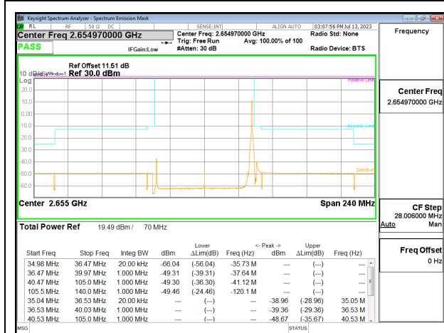
5G NR n41 70MHz QPSK High Channel RB1-187
