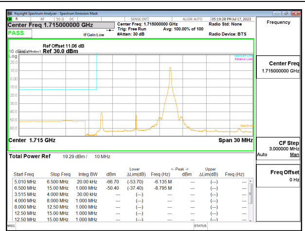
5G NR N66 10MHz QPSK LOW Ch RB1-50
