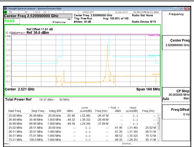
5G NR n41 50MHz QPSK Low Channel RB1-131
