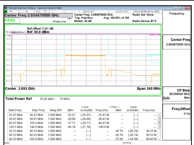
5G NR n41 70MHz QPSK High Channel RB180-0
