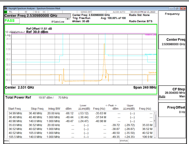
5G NR n41 70MHz QPSK Low Channel RB1-187
