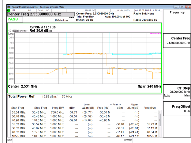
5G NR n41 70MHz QPSK Low Channel RB180-0
