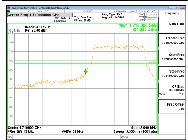
LTE66 1.4MHz QPSK LOW Ch RB6-0
