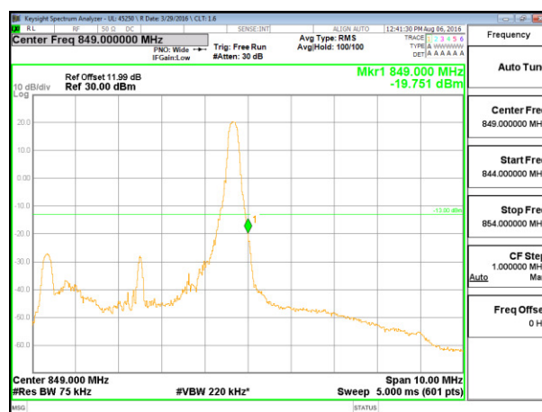
LTE B5 5MHz QPSK High Channel 1RB
