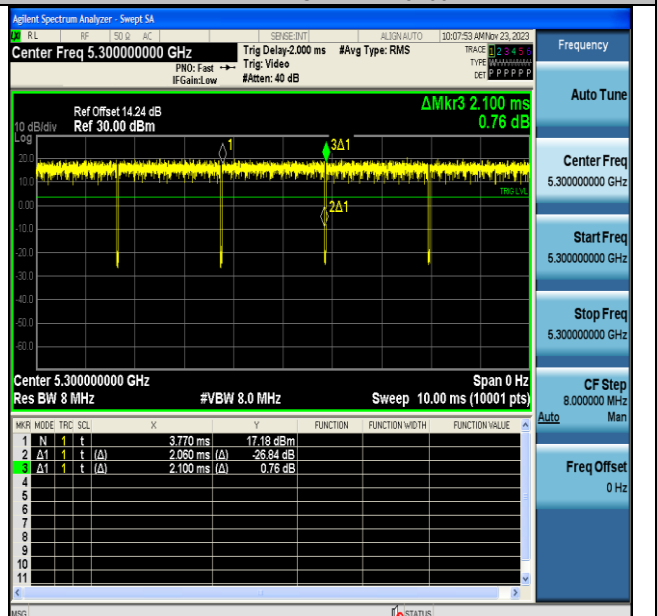
NTVN-11A-CDD-Ant7-5300
