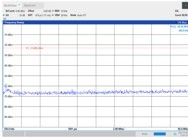
Band4-20MHz-QPSK-20050-1RB#0-Range2:0.15~30MHz
