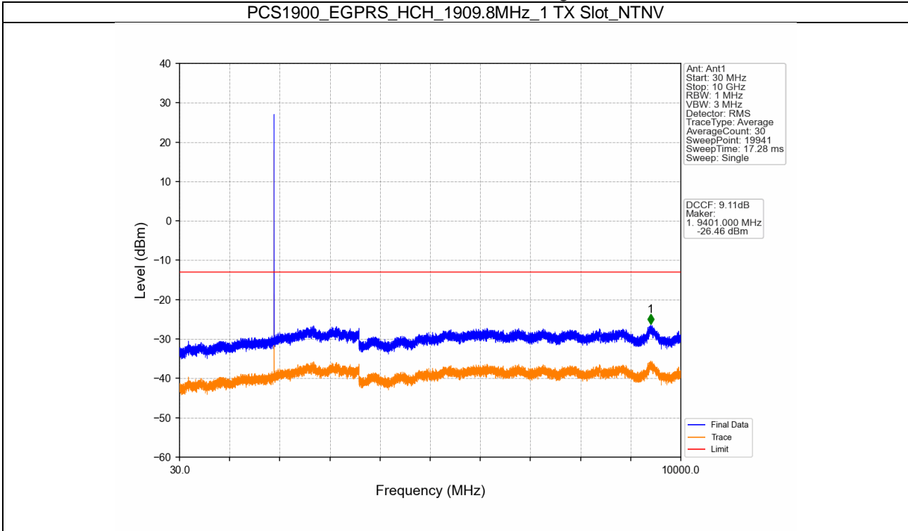
PCS1900_EGPRS_HCH_1909.8MHz_1 TX Slot_NTNV
