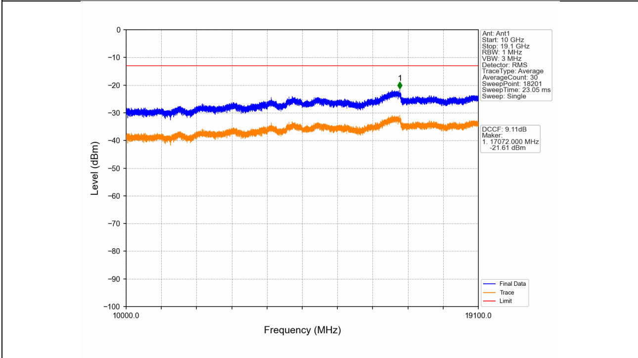
PCS1900_EGPRS_HCH_1909.8MHz_1 TX Slot_NTNV
