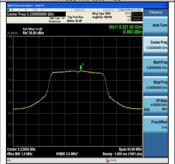
11A-CDD-Ant7-5320-PASS
