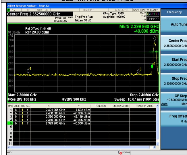
BLE 2M-Ant6-2402-PASS
