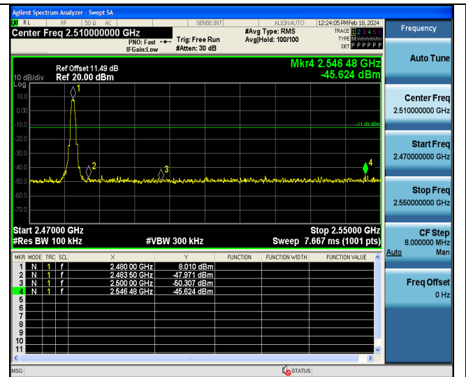
BLE 1M-Ant6-2480-PASS
