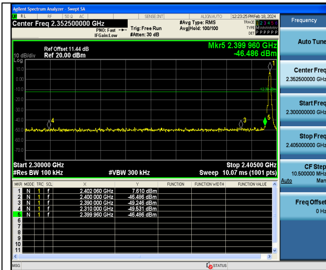
BLE 1M-Ant6-2402-PASS
