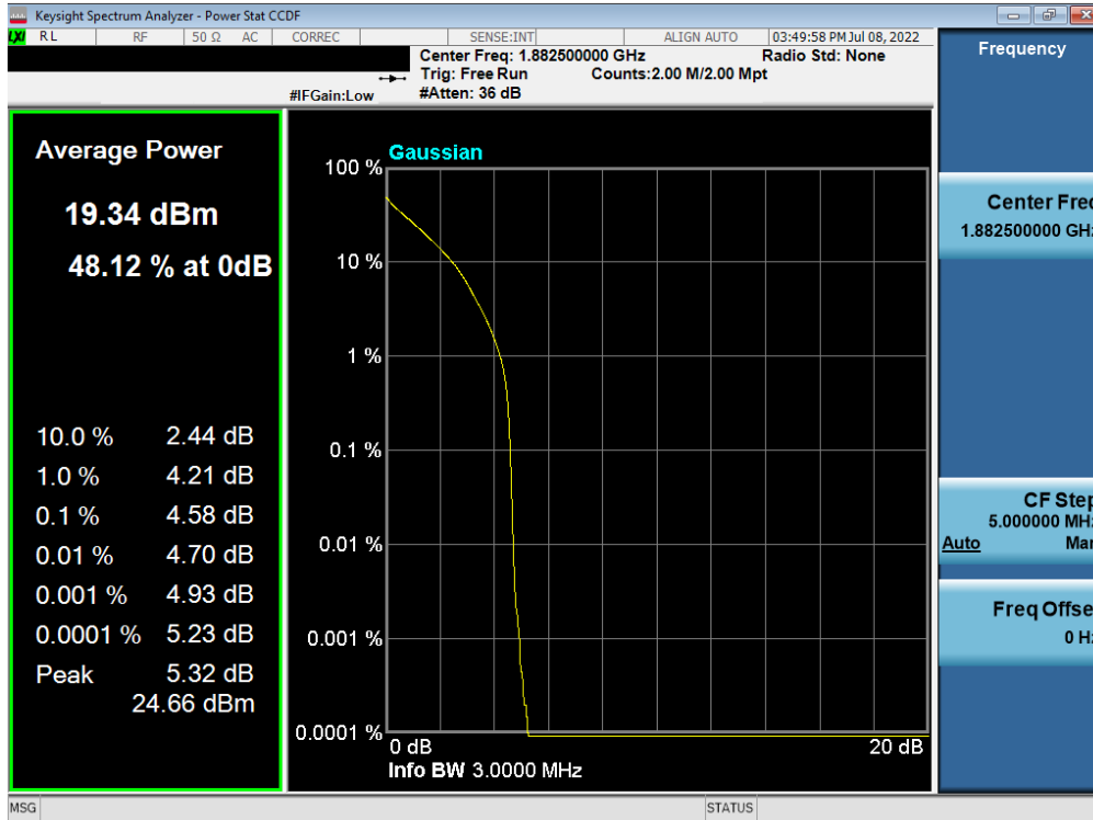
Plot 7-99. PAR Plot (LTE Band 25/2 - 3MHz QPSK - Full RB)
