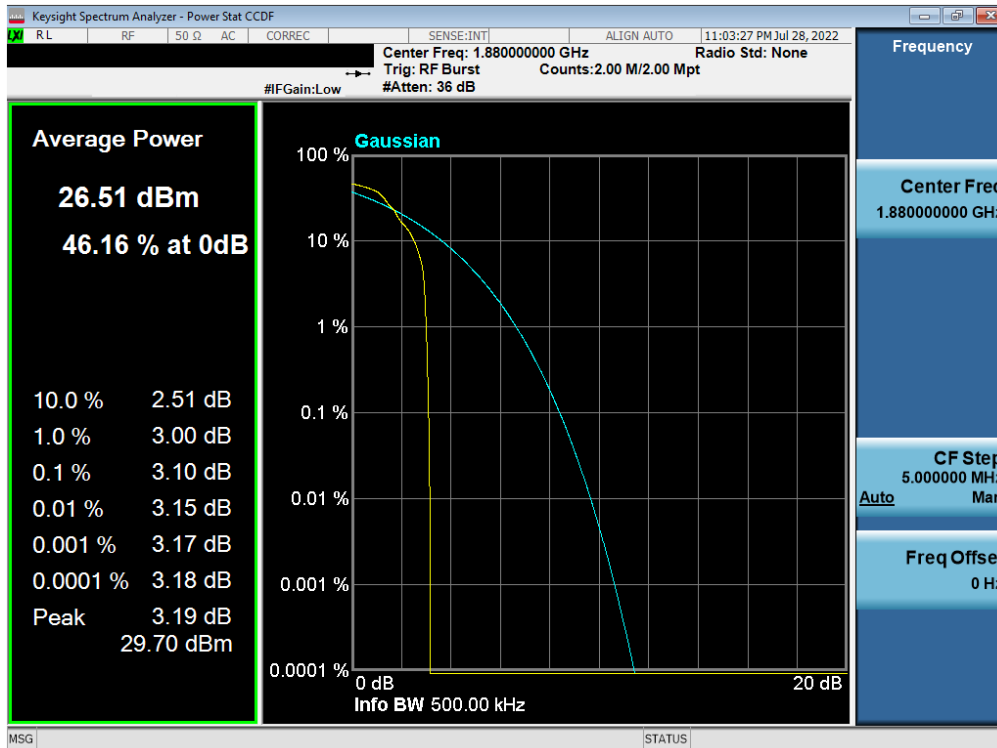
Plot 7-104. PAR Plot (EDGE, Ch. 661)
