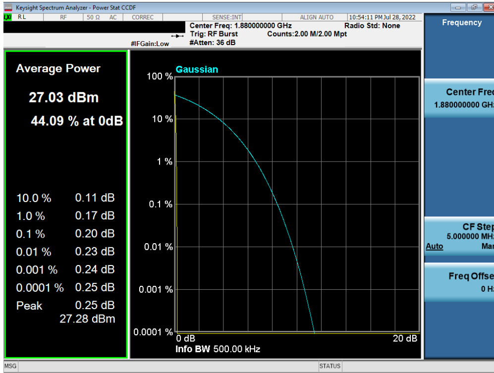
Plot 7-103. PAR Plot (GPRS, Ch. 661)
