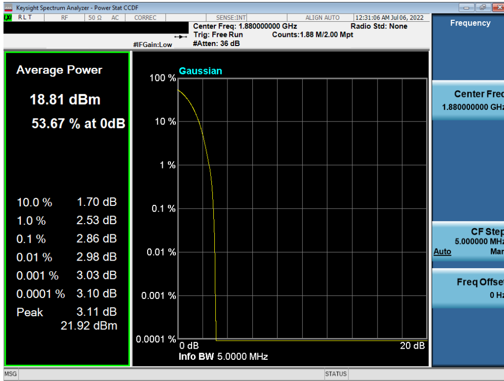
Plot 7-105. PAR Plot (WCDMA, Ch. 9400)
