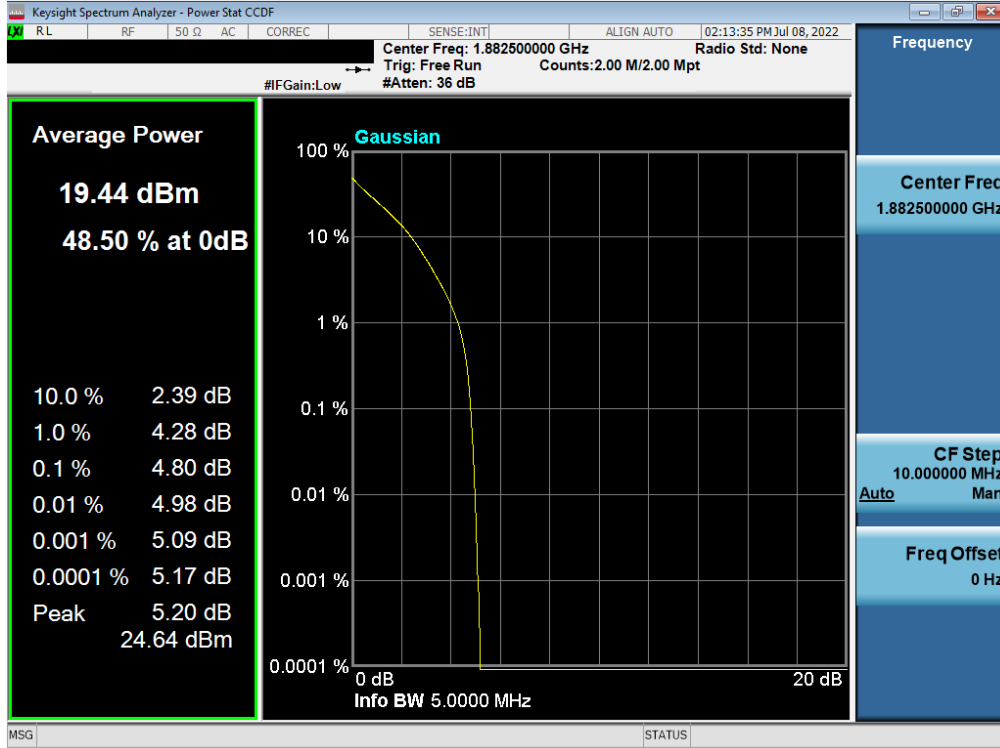
Plot 7-97. PAR Plot (LTE Band 25/2 - 5MHz QPSK - Full RB)
