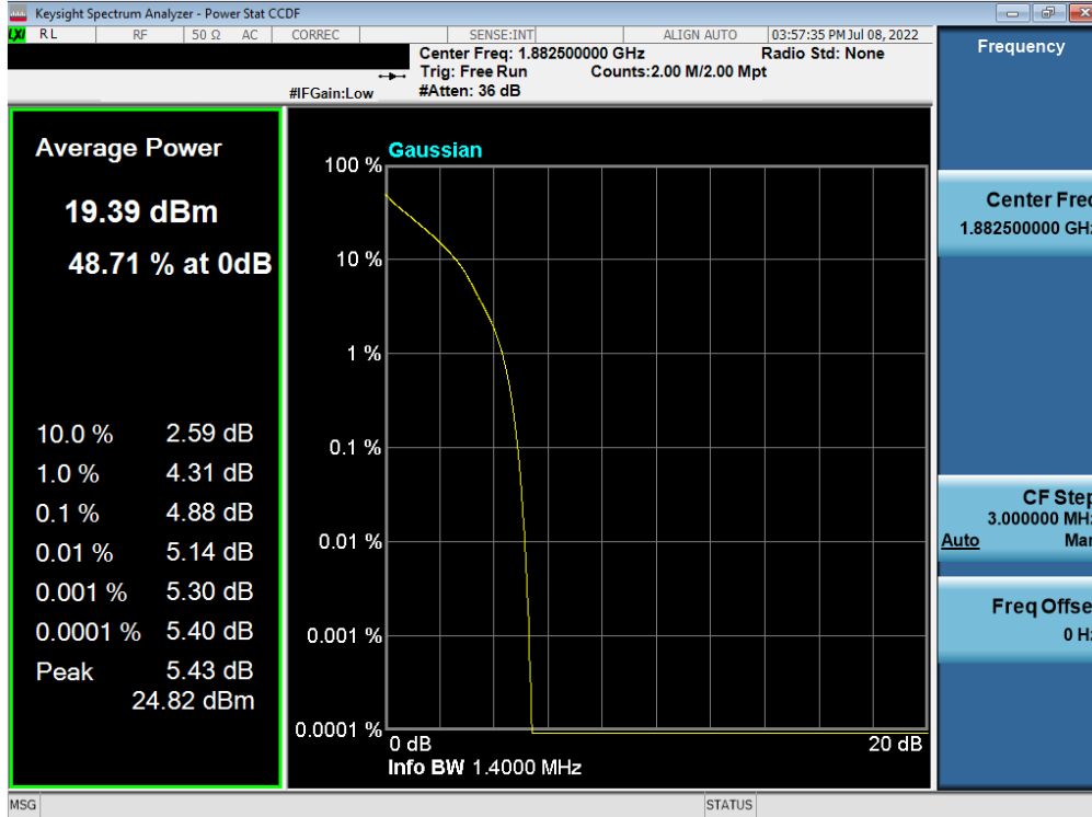
Plot 7-101. PAR Plot (LTE Band 25/2 - 1.4MHz QPSK - Full RB)
