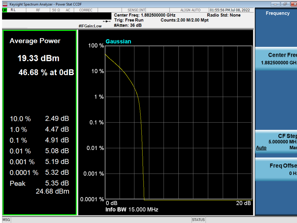
Plot 7-93. PAR Plot (LTE Band 25/2 - 15MHz QPSK - Full RB)
