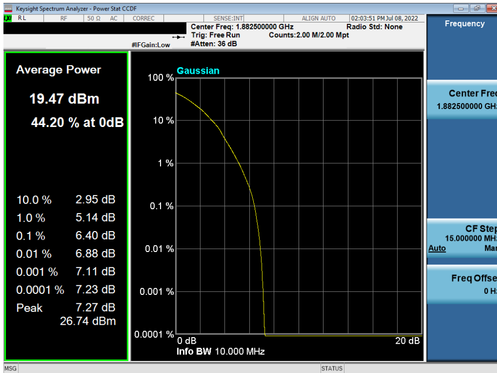
Plot 7-96. PAR Plot (LTE Band 25/2 - 10MHz 64-QAM - Full RB)
