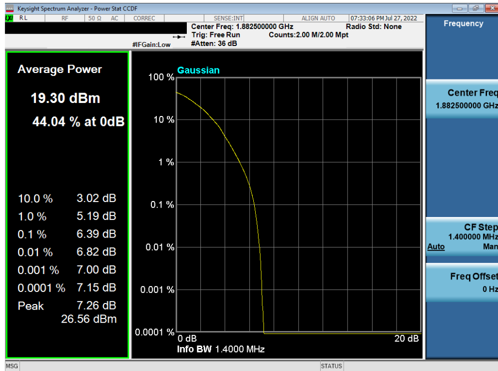
Plot 7-102. PAR Plot (LTE Band 25/2 - 1.4MHz 64-QAM - Full RB)
