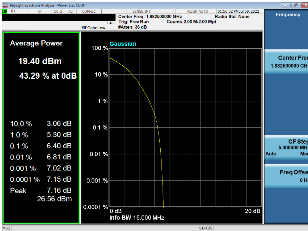
Plot 7-94. PAR Plot (LTE Band 25/2 - 15MHz 64-QAM - Full RB)
