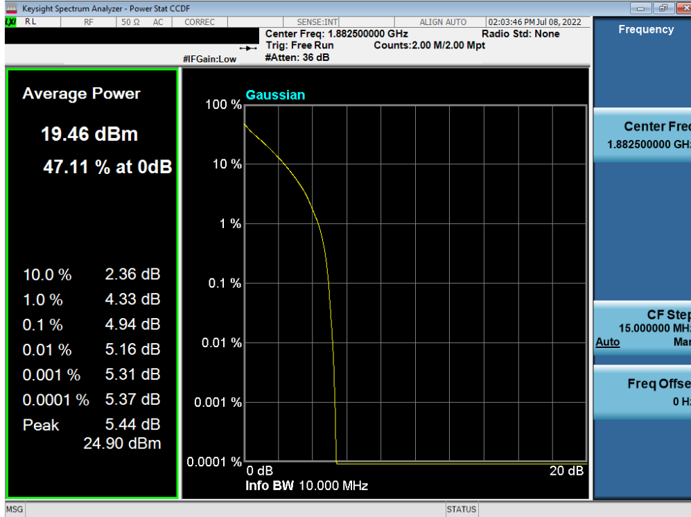
Plot 7-95. PAR Plot (LTE Band 25/2 - 10MHz QPSK - Full RB)
