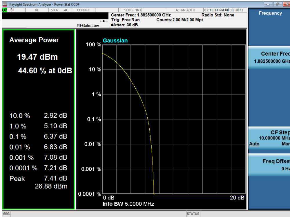
Plot 7-98. PAR Plot (LTE Band 25/2 - 5MHz 64-QAM - Full RB)
