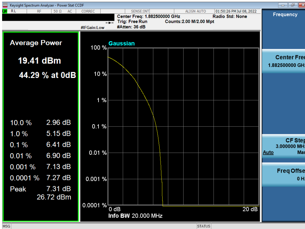
Plot 7-92. PAR Plot (LTE Band 25/2 - 20MHz 64-QAM - Full RB)
