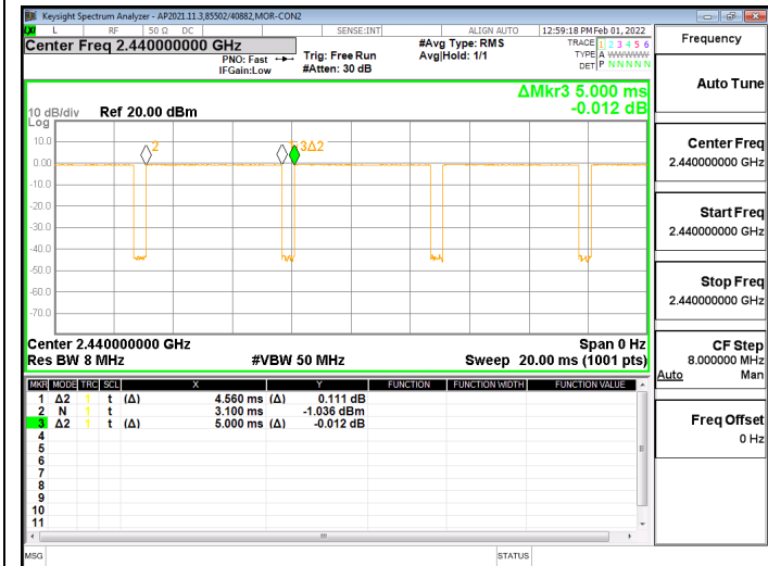
DUTY CYCLE BLE – 500Kbps CHAIN 0
