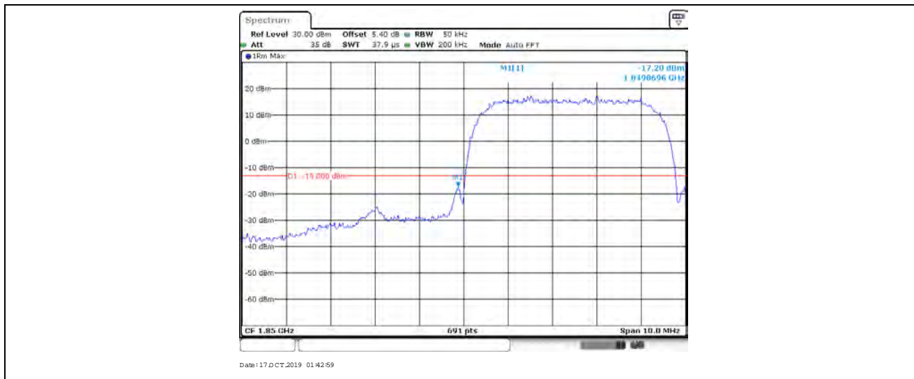
Band II_9262_QPSK
