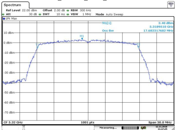
OBW_802.11n_HT20_5320MHz
