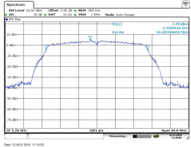
OBW_802.11a_5260MHz
