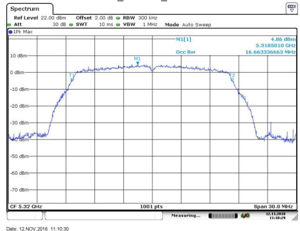
OBW_802.11a_5320MHz
