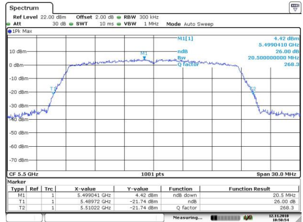
26dB_802.11n_HT20_5500MHz
