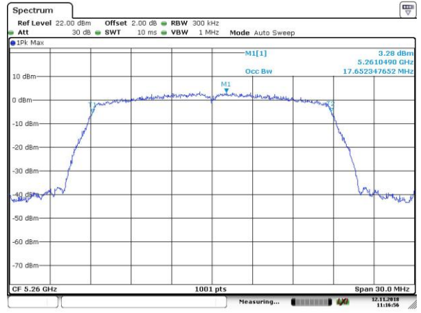
OBW_802.11n_HT20_5260MHz
