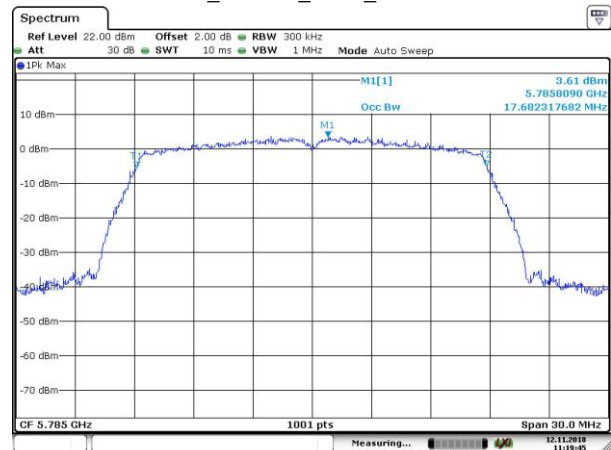
OBW_802.11n_HT20_5785MHz
