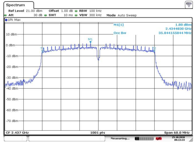
obw_802.11n_40MHz_Chain0_2437MHz
