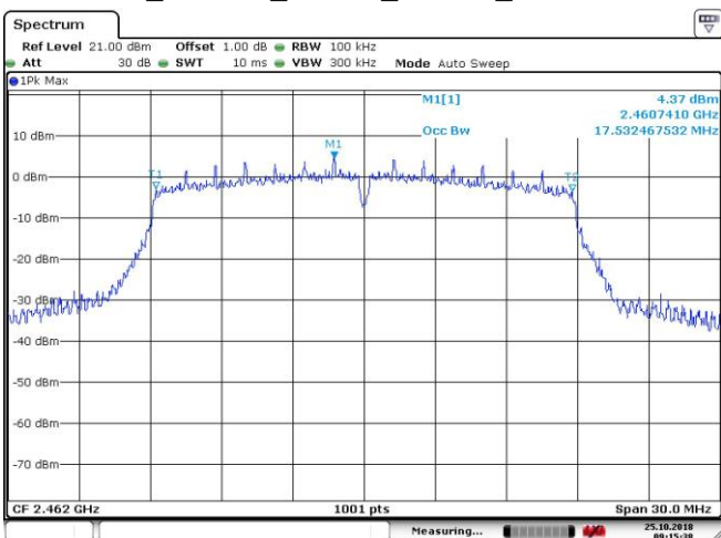
obw_802.11n_20MHz_Chain0_2462MHz
