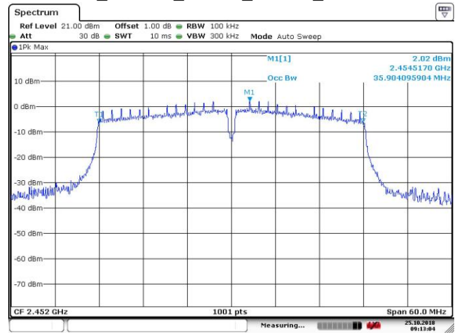
obw_802.11n_40MHz_Chain0_2452MHz
