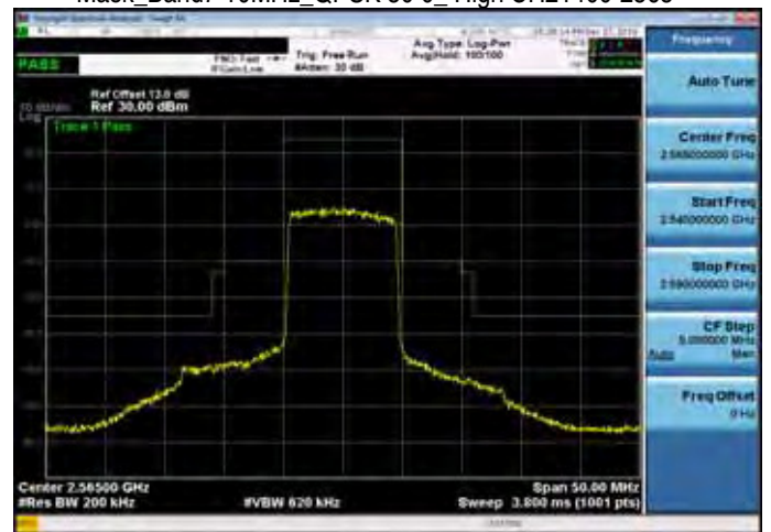
Mask_Band7 10MHz_QPSK 50 0_High CH21400-2565
