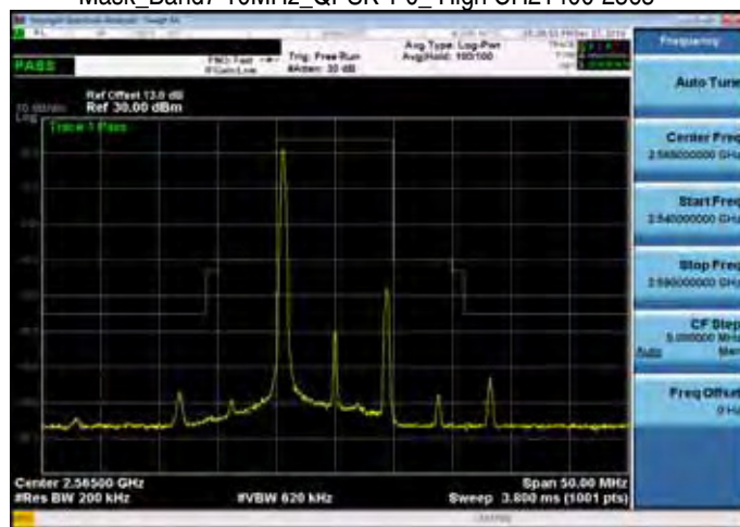
Mask_Band7 10MHz_QPSK 1 0_High CH21400-2565
