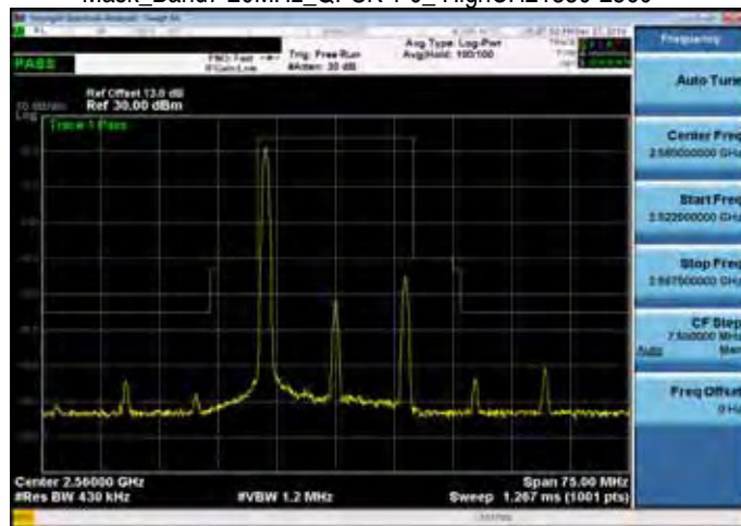
Mask_Band7 20MHz_QPSK 1 0_HighCH21350-2560
