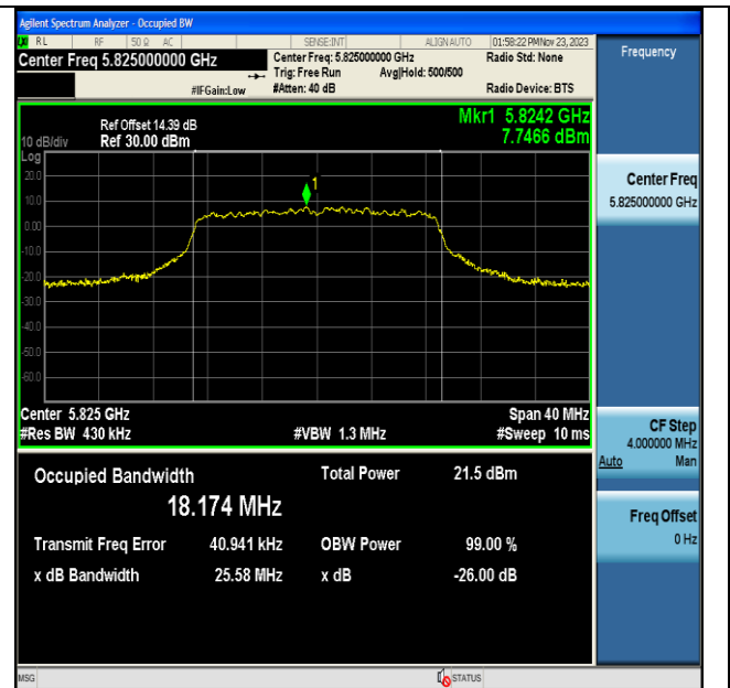
11N20MIMO-Ant7-5825
