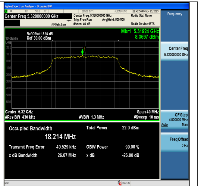
11N20MIMO-Ant7-5320
