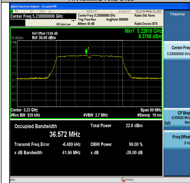
11N40MIMO-Ant6-5230
