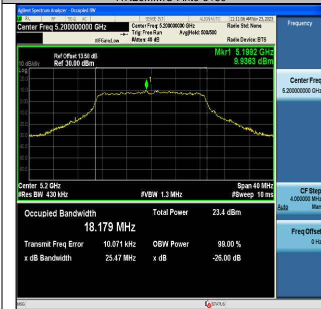
11N20MIMO-Ant6-5200
