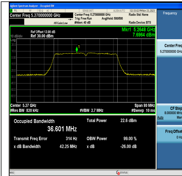
11N40MIMO-Ant6-5270
