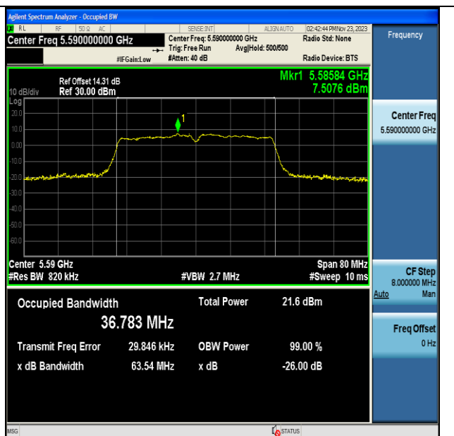
11N40MIMO-Ant7-5590
