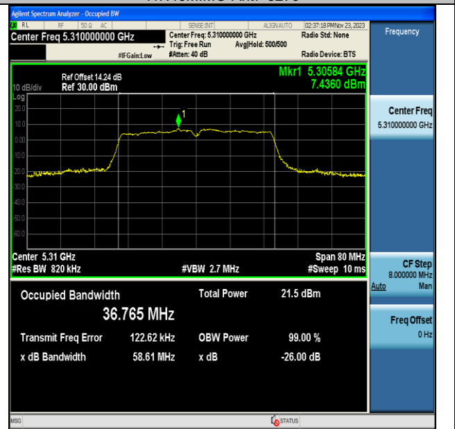
11N40MIMO-Ant7-5310
