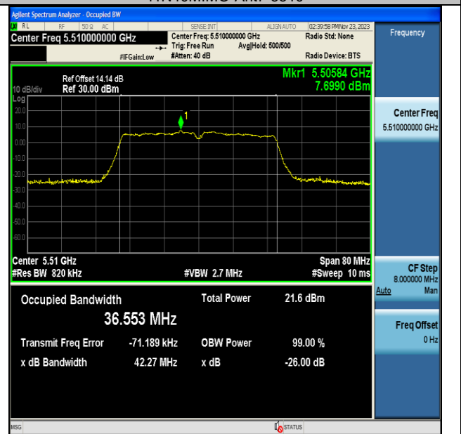
11N40MIMO-Ant7-5510
