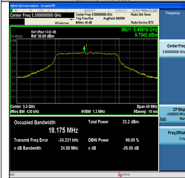
11N20MIMO-Ant6-5500
