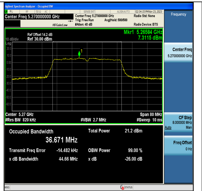
11N40MIMO-Ant7-5270
