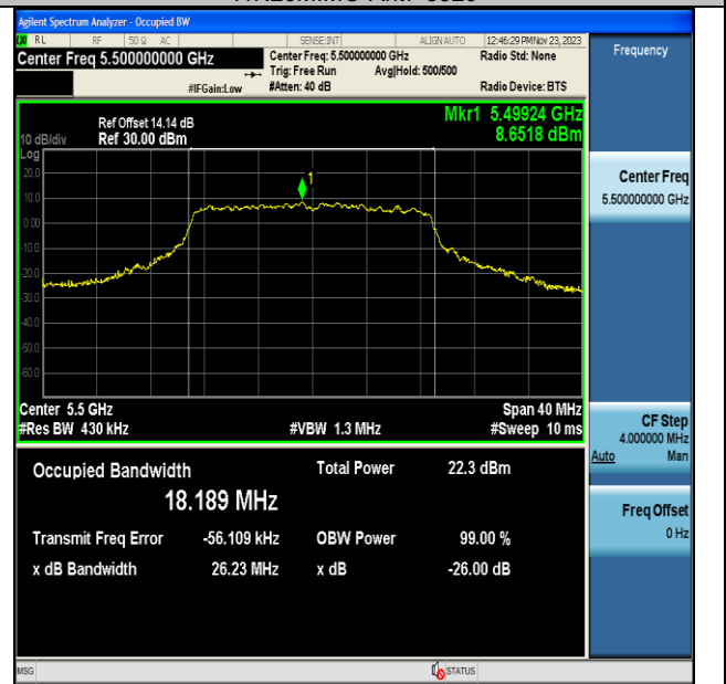
11N20MIMO-Ant7-5500
