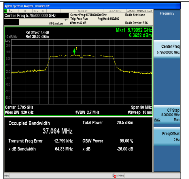
11N40MIMO-Ant7-5795
