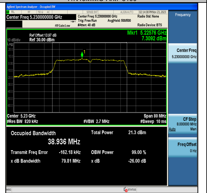
11N40MIMO-Ant7-5230
