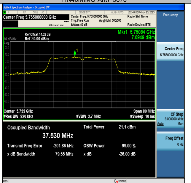
11N40MIMO-Ant7-5755
