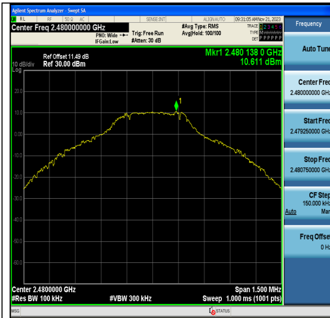
DH5-Ant6-2480-0-Reference-PASS
