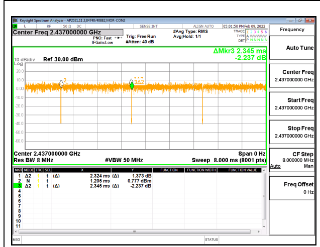
802.11ax HE20 OFDMA, RU index 52T MODE,2TX
