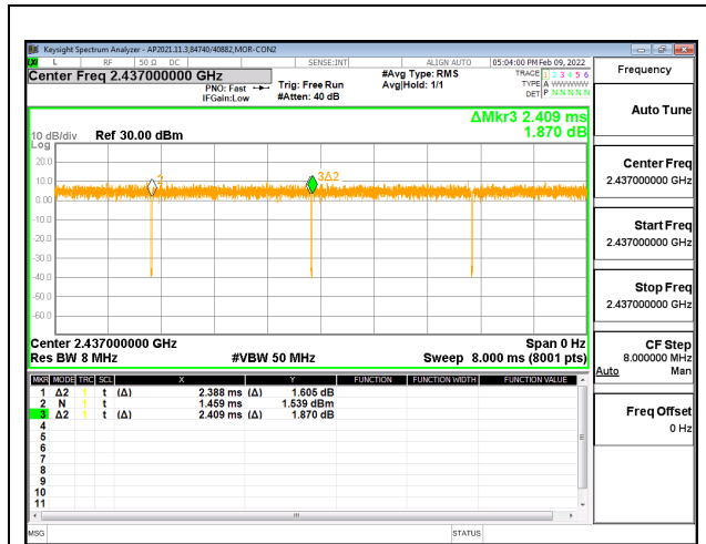
802.11ax HE20 OFDMA, RU index 242T MODE,2TX
