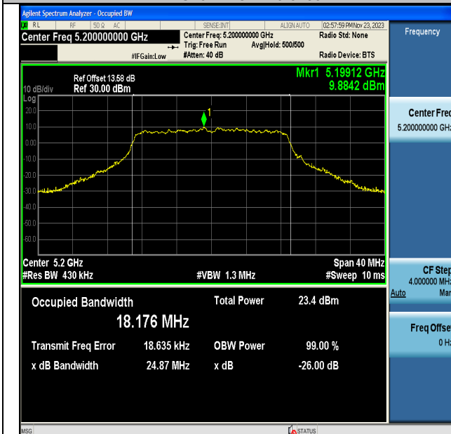
11A20MIMO-Ant6-5200
