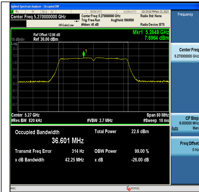
11N40MIMO-Ant6-5270
