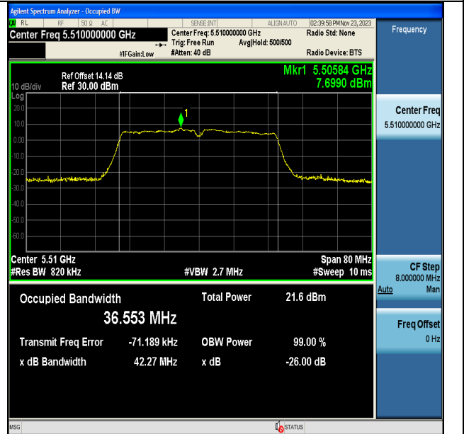
11N40MIMO-Ant7-5510
