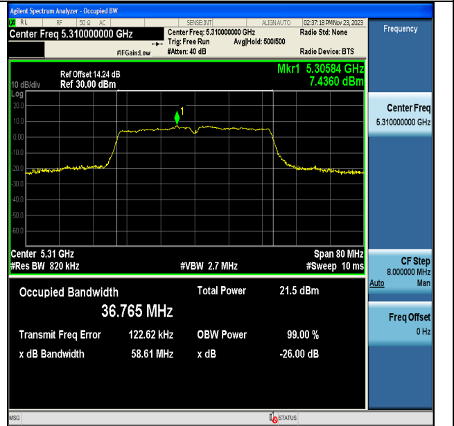
11N40MIMO-Ant7-5310
