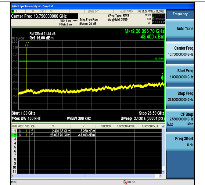
BLE 2M-Ant6-2402-1000~26500-PASS
