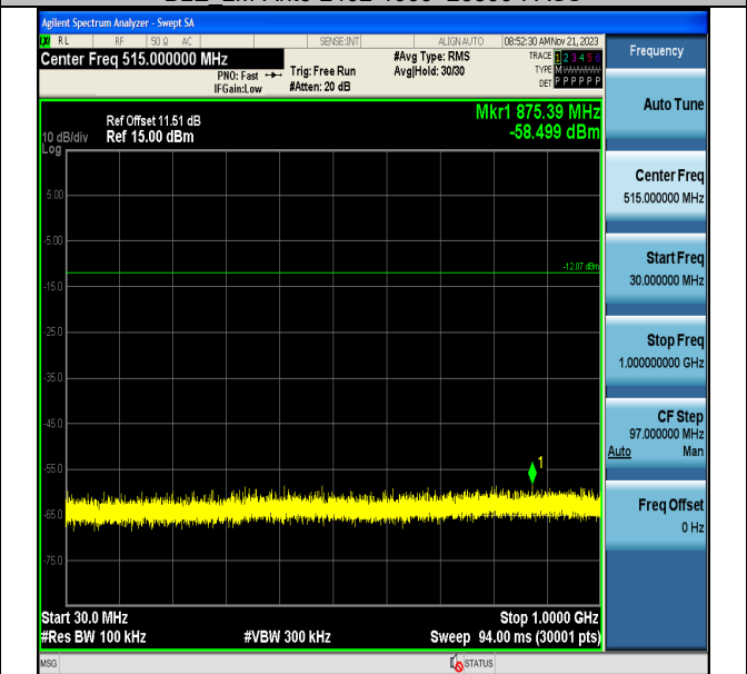
BLE 2M-Ant6-2440-30~1000-PASS
