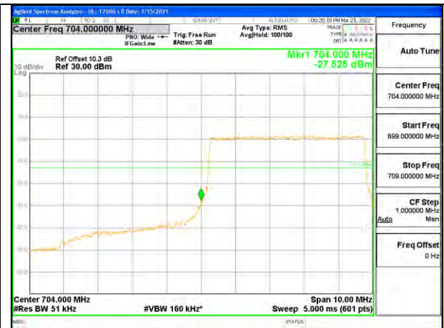
LTE17 5MHz QPSK LOW Ch RB25-0
