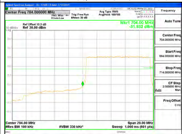
LTE17 10MHz QPSK LOW Ch RB50-0
