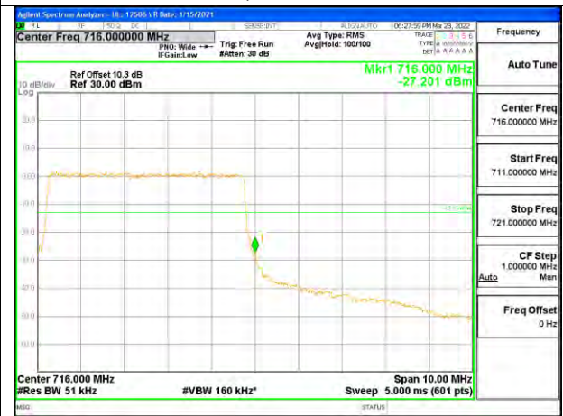
LTE17 5MHz QPSK HIGH Ch RB25-0
