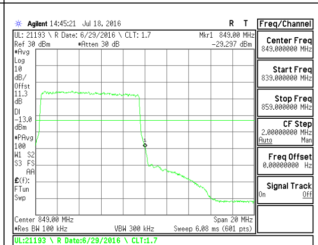
LTE B5 10MHz QPSK High Channel 1RB
