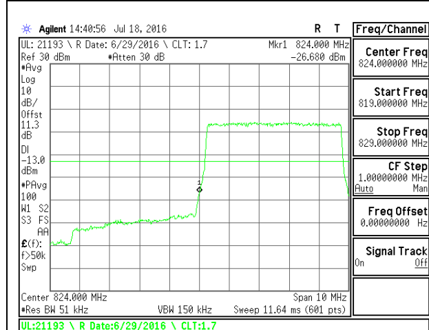
LTE B5 5MHz QPSK Low Channel 1RB
