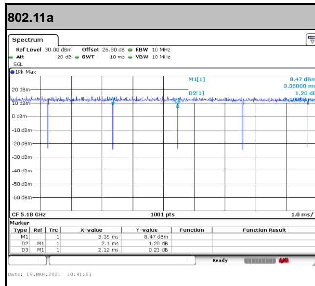
MIMO <Chain 1>
