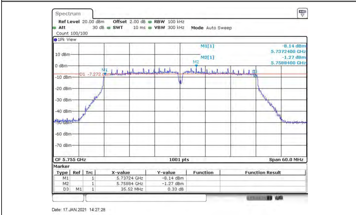
11N40MIMO_ANT6_5755
