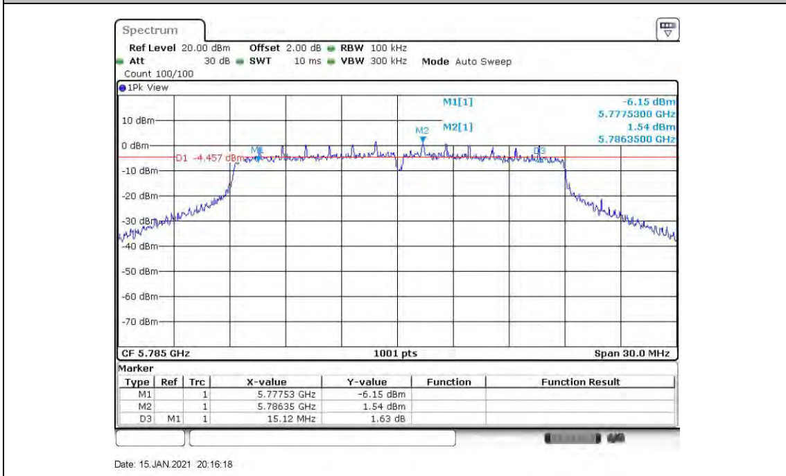
11AC20MIMO_ANT6_5785
