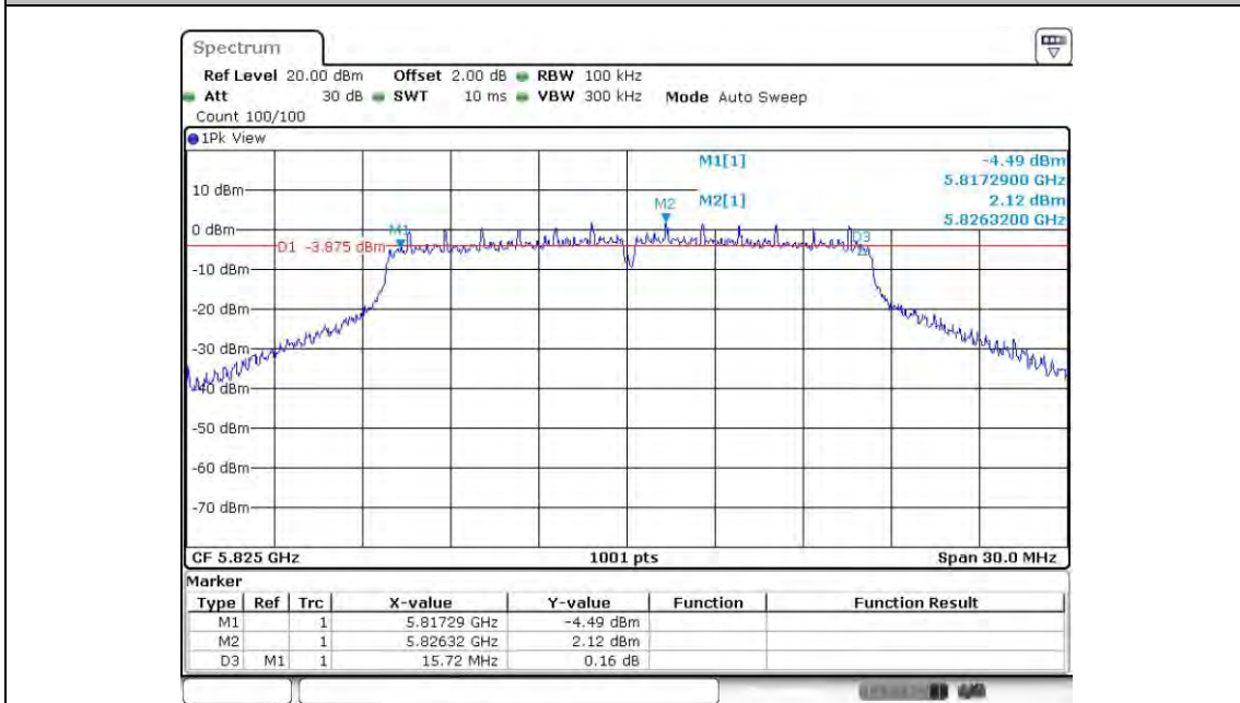
11A_ANT6_5825
