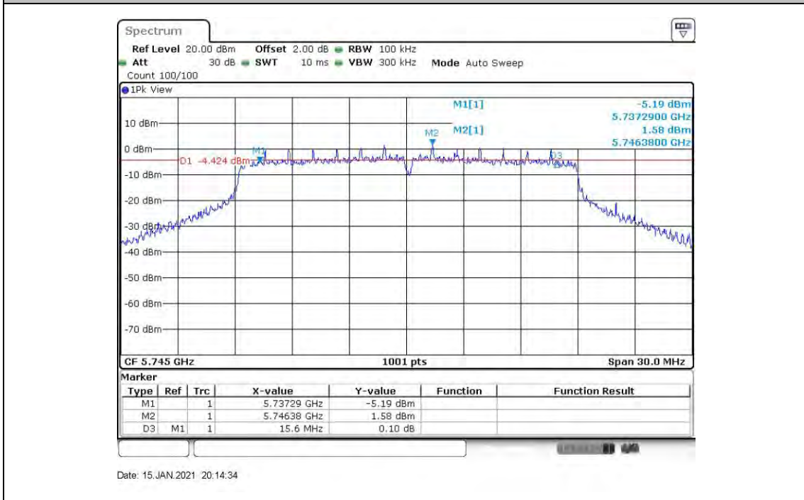
11AC20MIMO_ANT7_5745
