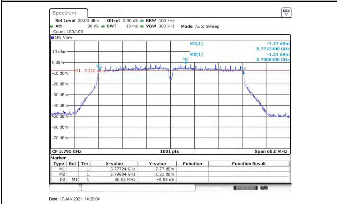
11N40MIMO_ANT6_5795
