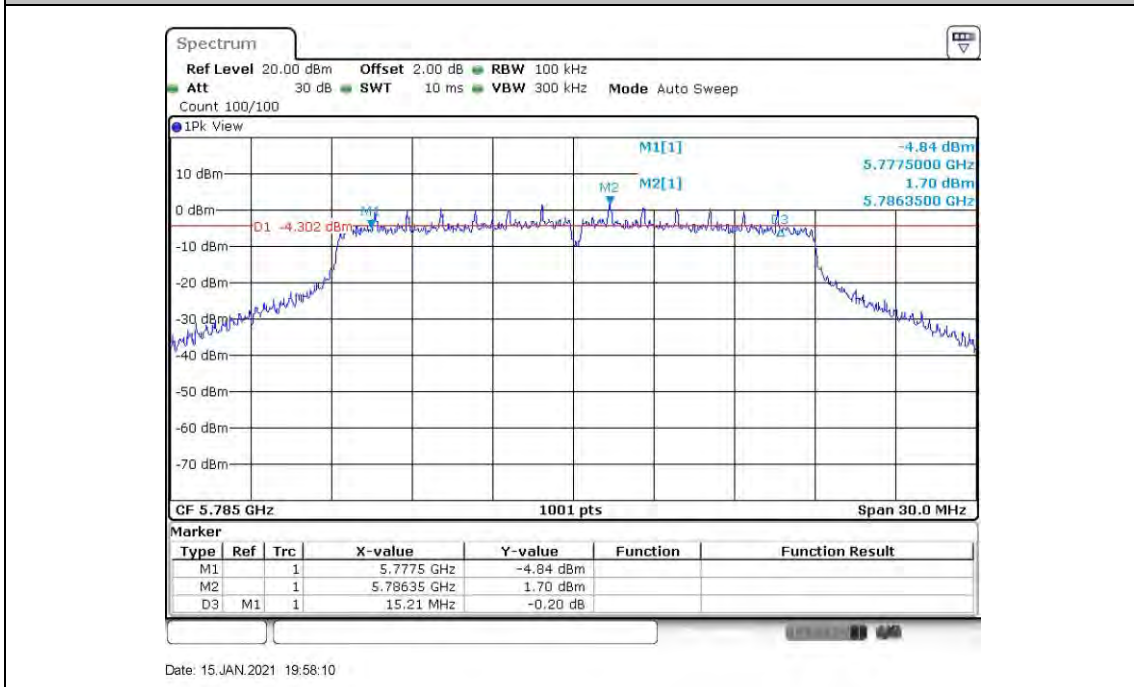
11N20MIMO_ANT6_5785
