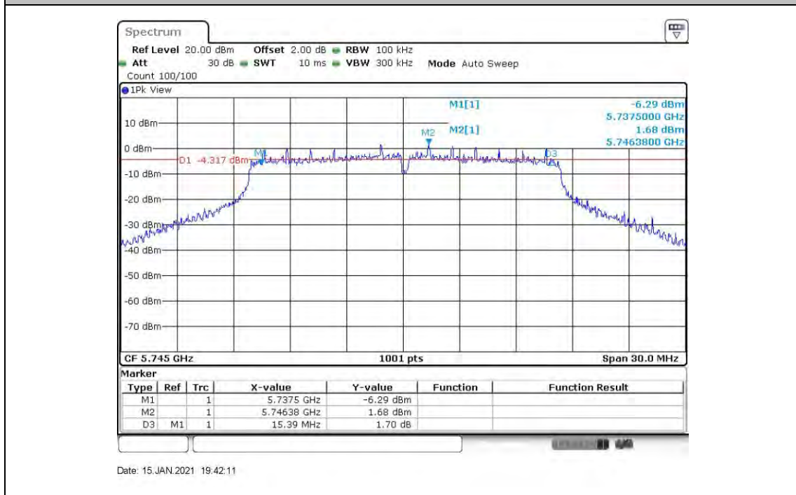
11A-CDD_ANT7_5745
