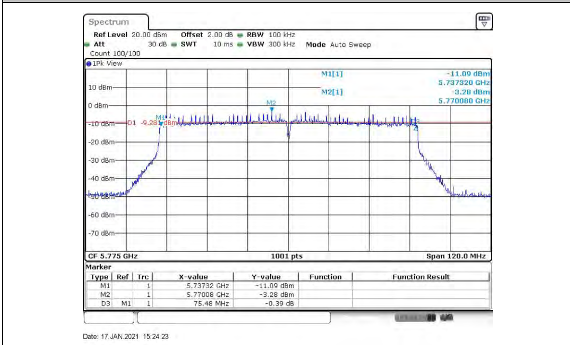
11AC80MIMO_ANT6_5775
