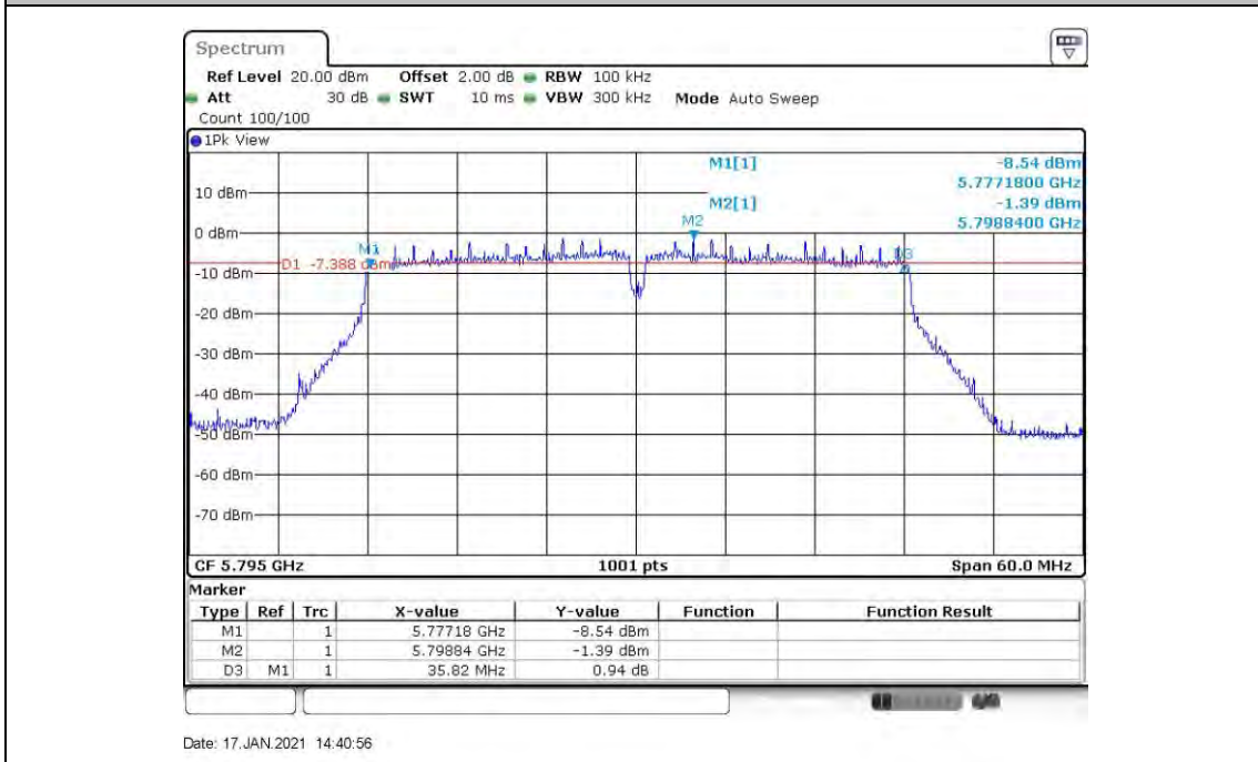
11AC40MIMO_ANT6_5795
