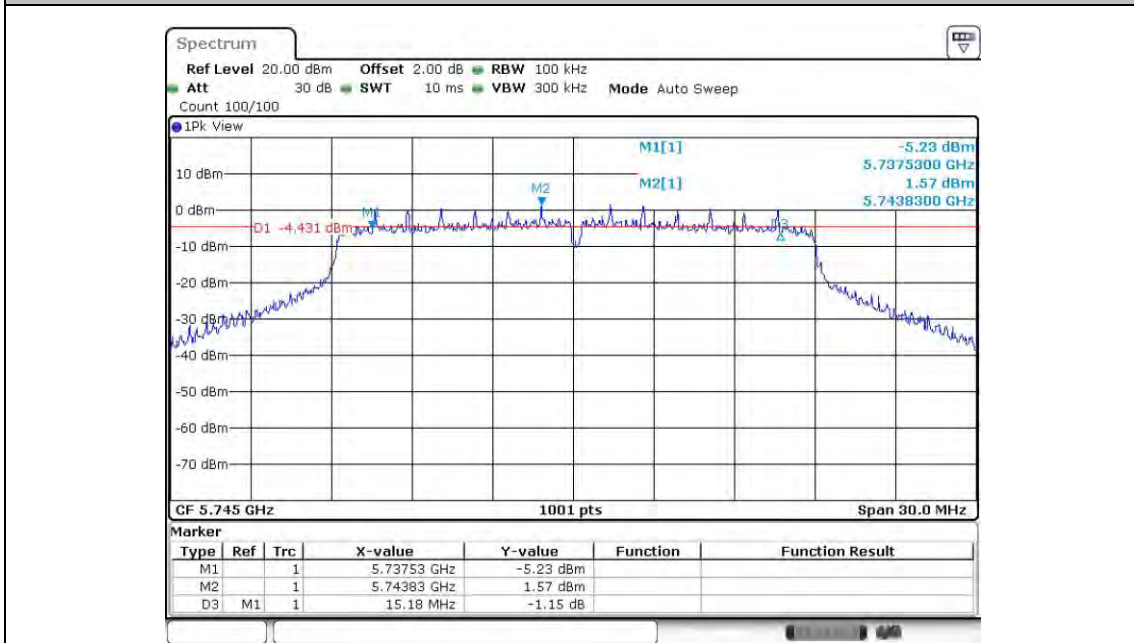
11N20MIMO_ANT6_5745
