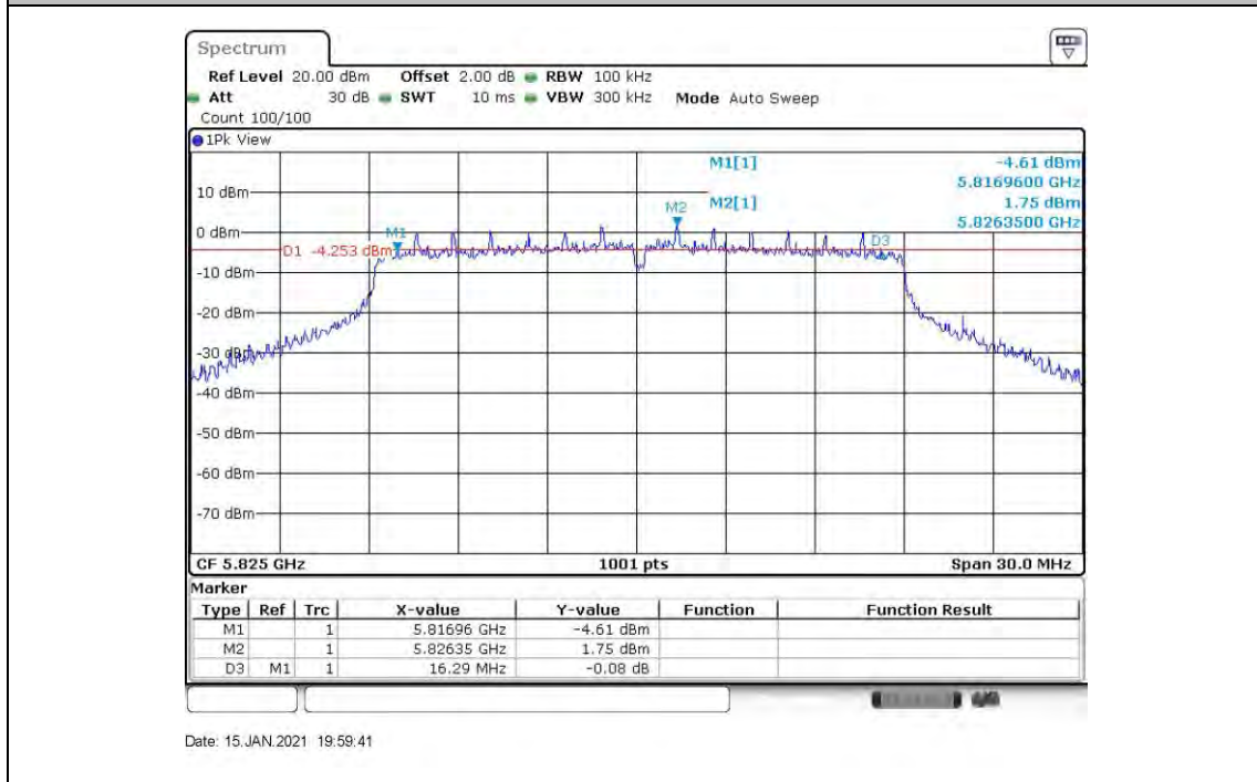
11N20MIMO_ANT7_5825
