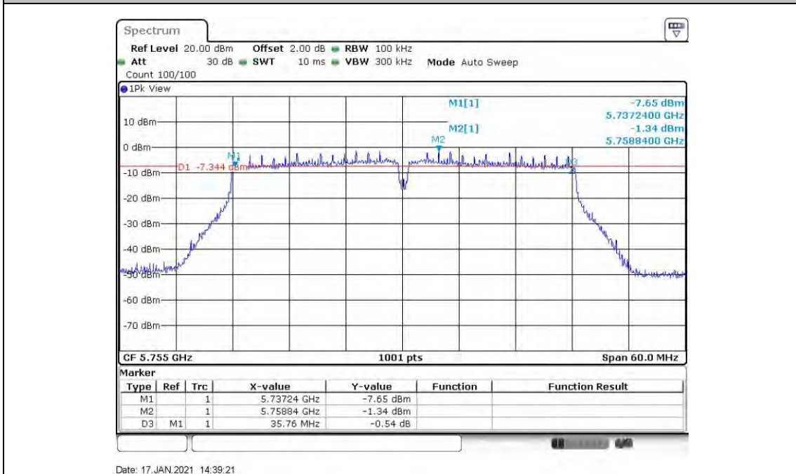
11AC40MIMO_ANT6_5755
