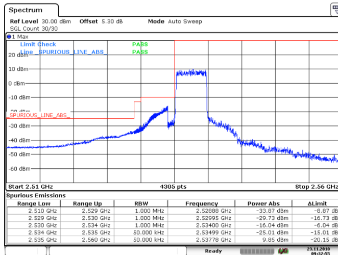
Band41_5MHz_QPSK_40065_25RB#0
