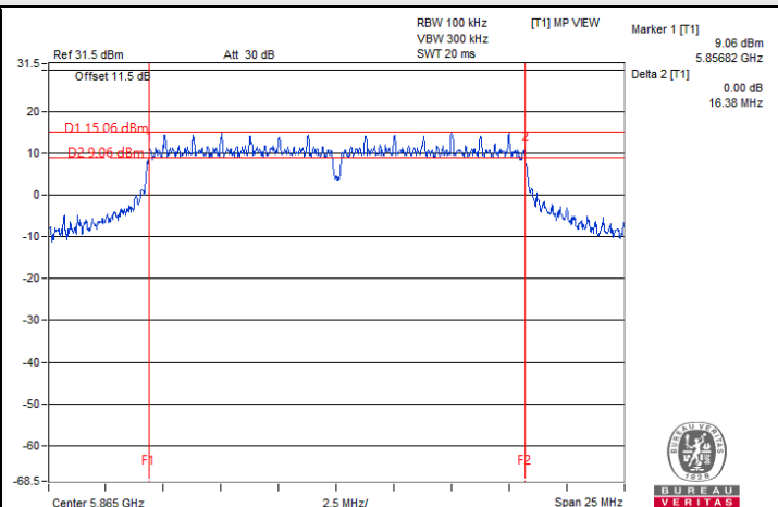
802.11be (EHT20) Beamforming / Chain 0 : CH 173
