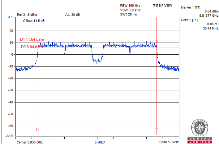
802.11be (EHT40) Beamforming / Chain 0 : CH 167
