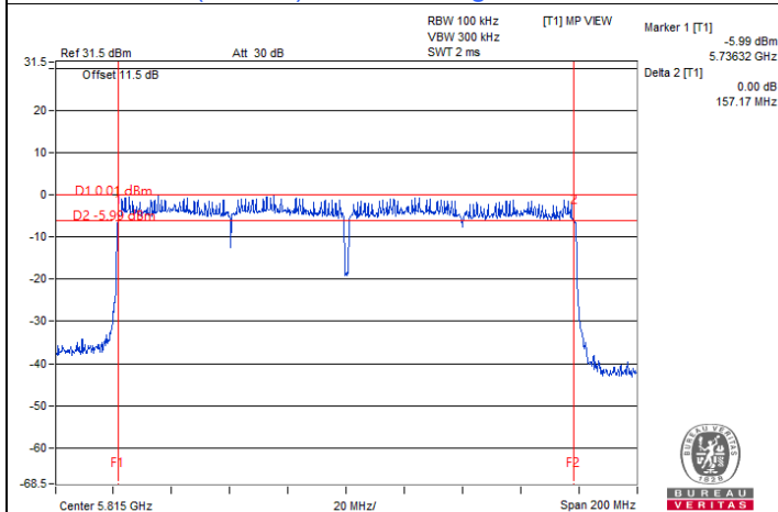
802.11be (EHT160) Beamforming / Chain 0 : CH 163
