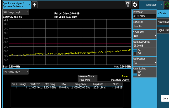
1RB CH 38725 (2307.5 MHz)
