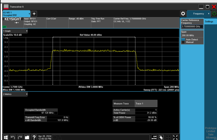
QPSK CH 650000 (3750 MHz)
