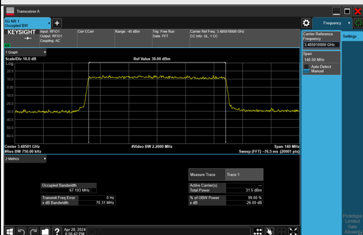
QPSK CH 632334 (3485.01 MHz)
