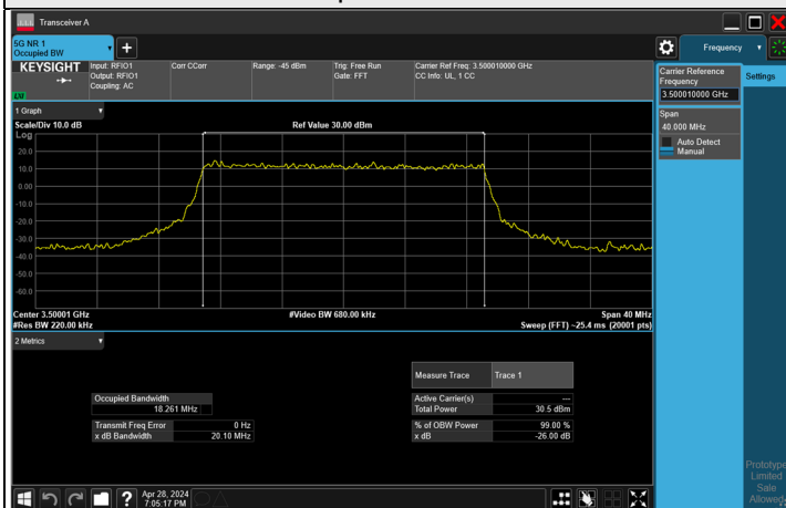
16QAM CH 633334 (3500.01 MHz)
