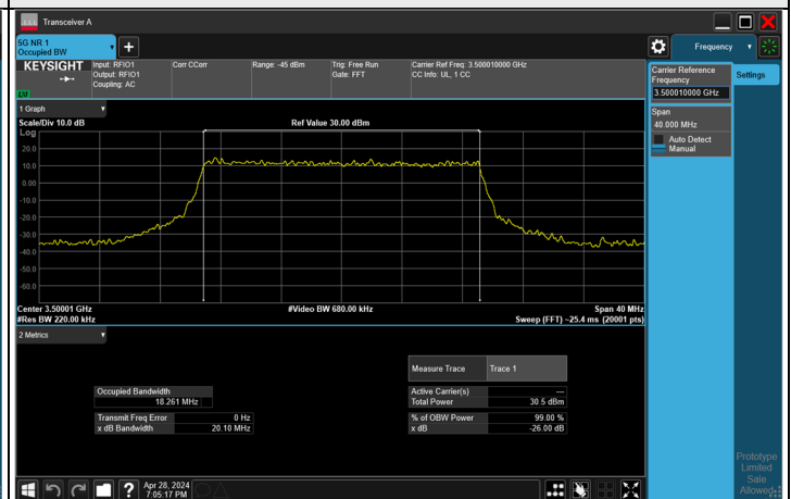
16QAM CH 633334 (3500.01 MHz)
