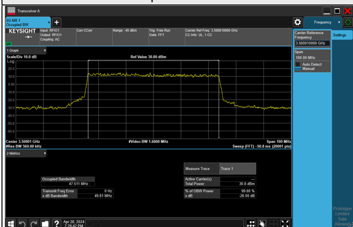
64QAM CH 633334 (3500.01 MHz)
