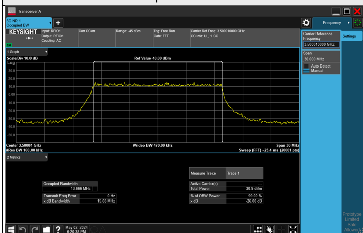
QPSK CH 633334 (3500.01 MHz)
