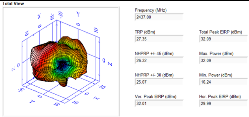
2.4GHz_EHT20_CH6_BF On Nss1
