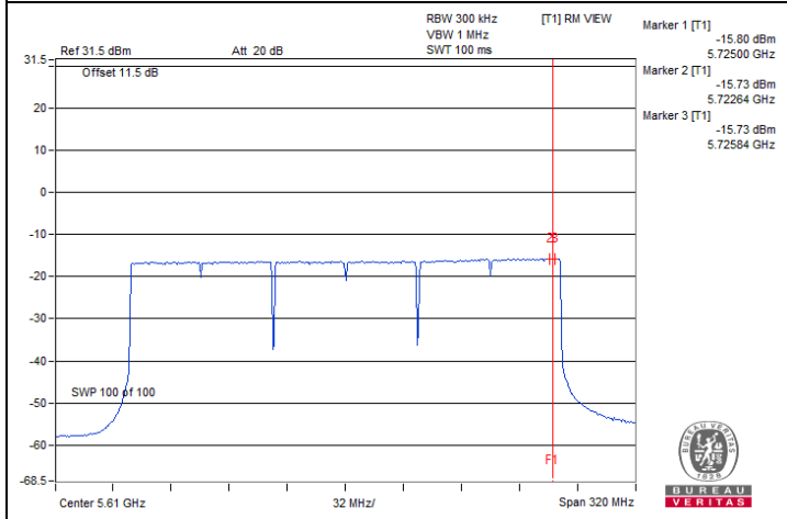
802.11be (EHT240) / Chain 0 : CH 122 (U-NII-3)
