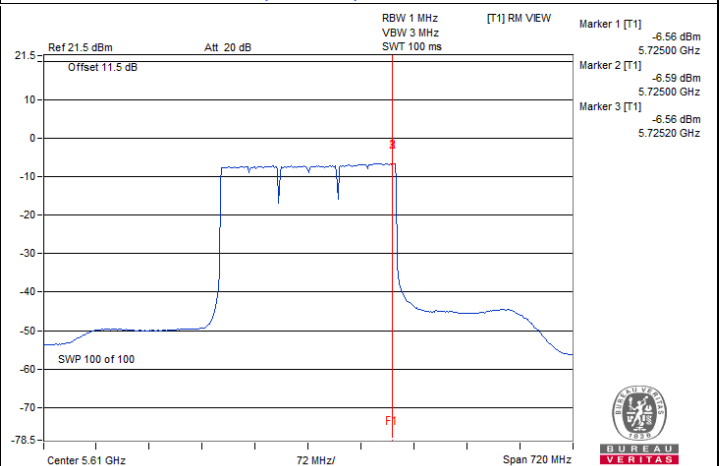
802.11be (EHT240) / Chain 0 : CH 122 (U-NII-2C)
