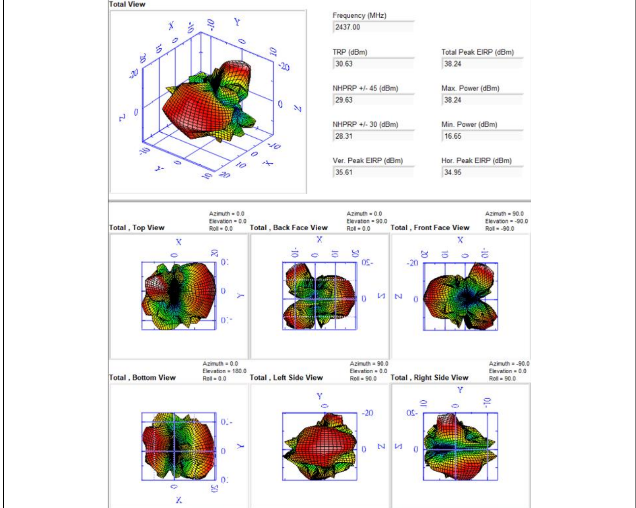
2.4GHz_EHT20_CH6_BF On Nss1
