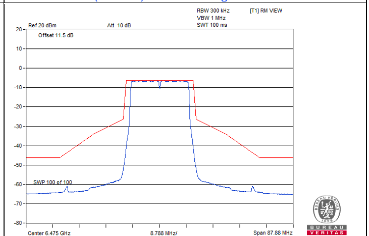
802.11be (EHT20) Beamforming / Chain 1 : CH 105
