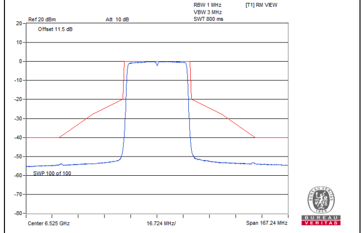
802.11be (EHT40) Beamforming / Chain 0 : CH 115
