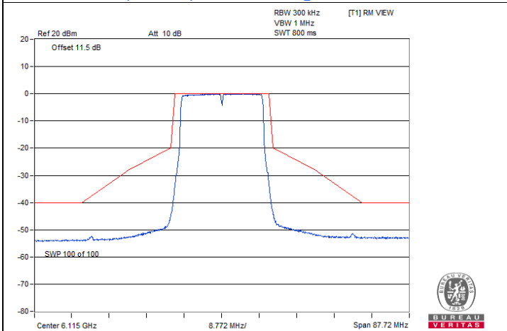
802.11be (EHT20) Beamforming / Chain 2 : CH 33
