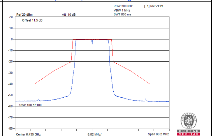
802.11be (EHT20) Beamforming / Chain 2 : CH 97
