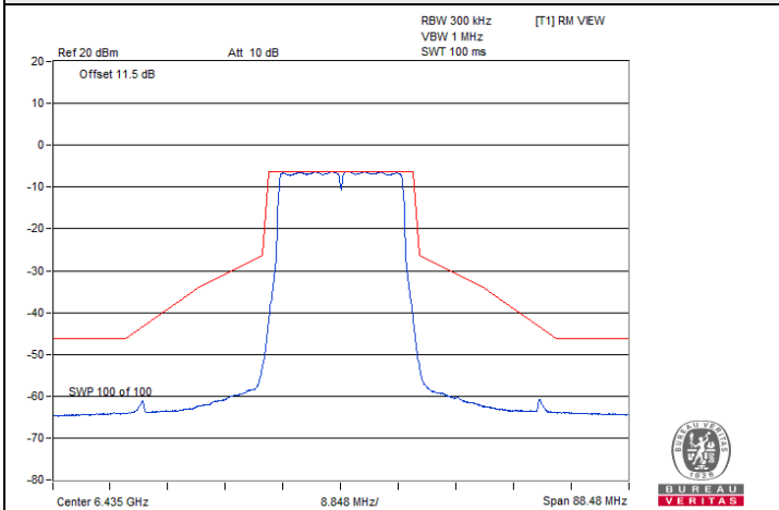
802.11be (EHT20) Beamforming / Chain 3 : CH 97
