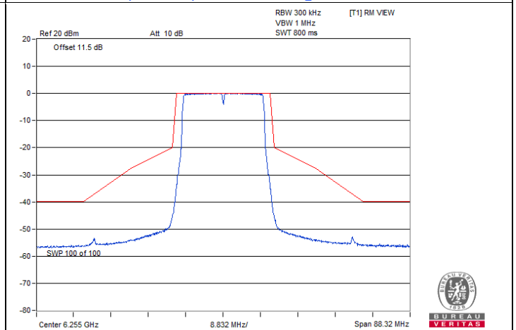
802.11be (EHT20) Beamforming / Chain 2 : CH 61
