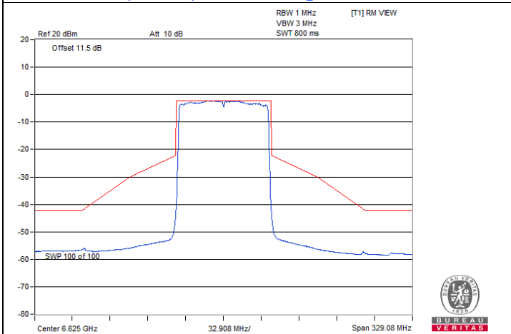
802.11be (EHT80) Beamforming / Chain 3 : CH 135
