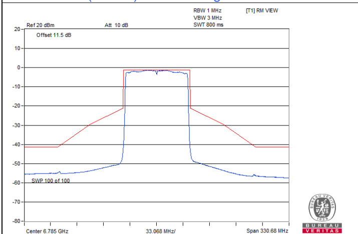
802.11be (EHT80) Beamforming / Chain 3 : CH 167
