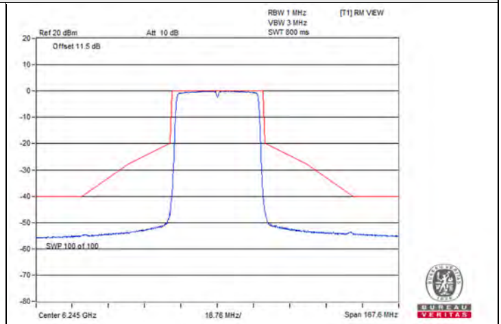
802.11be (EHT40) Beamforming / Chain 0 : CH 59
