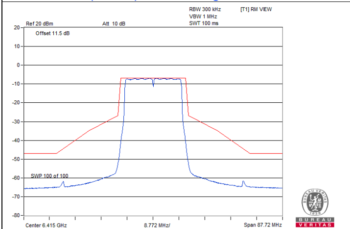
802.11be (EHT20) Beamforming / Chain 2 : CH 93
