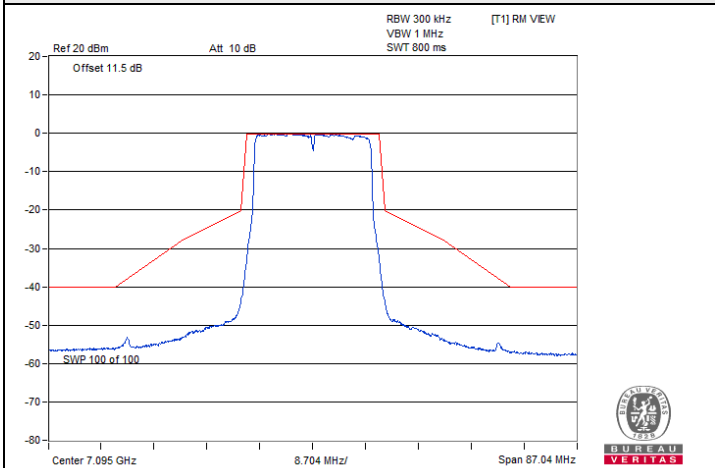
802.11be (EHT20) Beamforming / Chain 1 : CH 229
