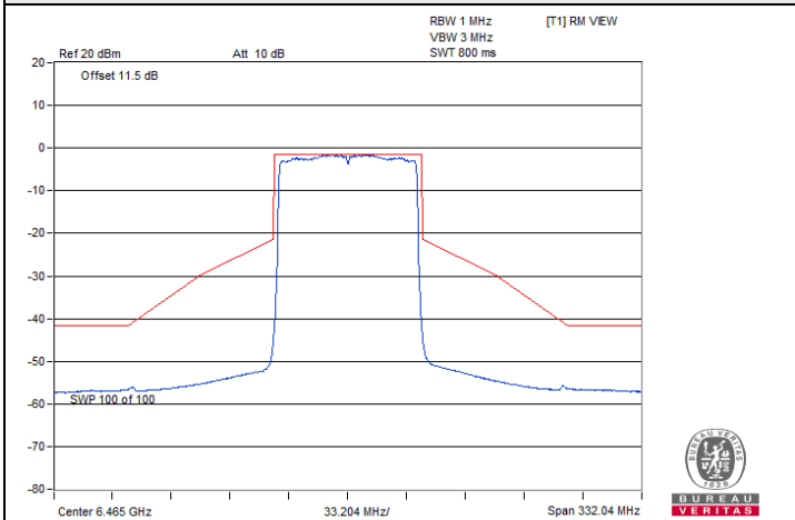
802.11be (EHT80) Beamforming / Chain 3 : CH 103
