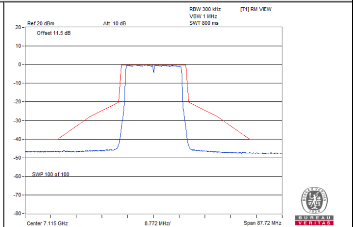
802.11be (EHT20) Beamforming / Chain 1 : CH 233
