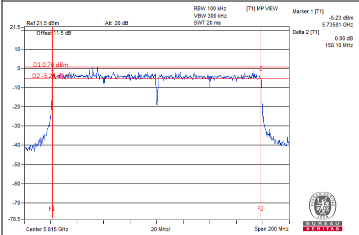
802.11be (EHT160) / Chain 3 : CH 163
