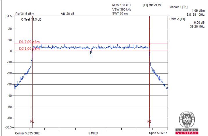
802.11be (EHT40) / Chain 3 : CH 167
