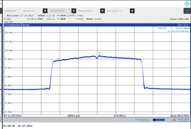
802.11ax (HE40)
