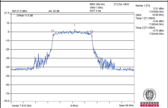
802.11ax (HE20)_Chain 0 / CH 213 (U-NII-8 Band)
