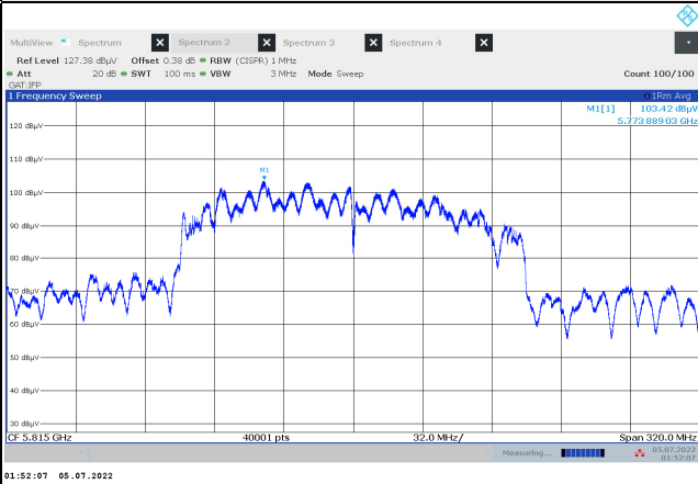
802.11ax (HE160)
