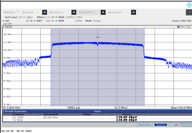
802.11ax (HE80)
