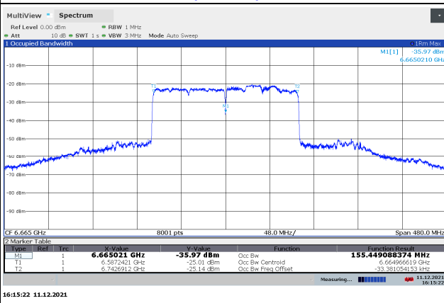
802.11ax (HE160) / CH 143
