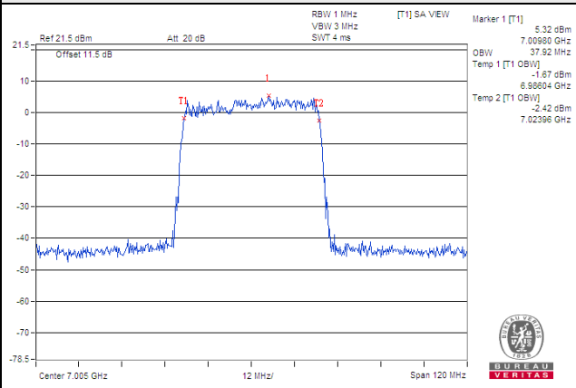
802.11ax (HE40)_Chain 0 / CH 211 (U-NII-8 Band)
