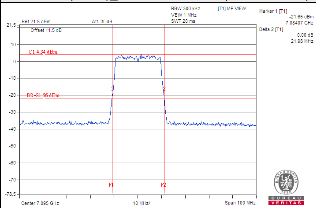
802.11ax (HE20)_Chain 1 / CH 229 (U-NII-8 Band)
