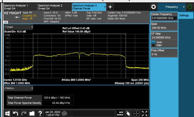
802.11ax (HE160)
