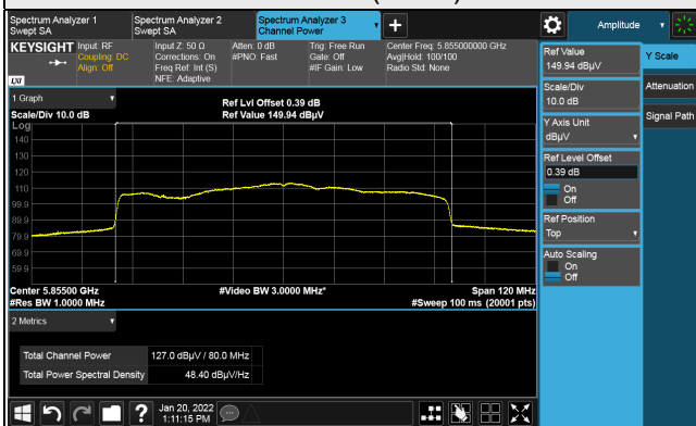
802.11ax (HE80)
