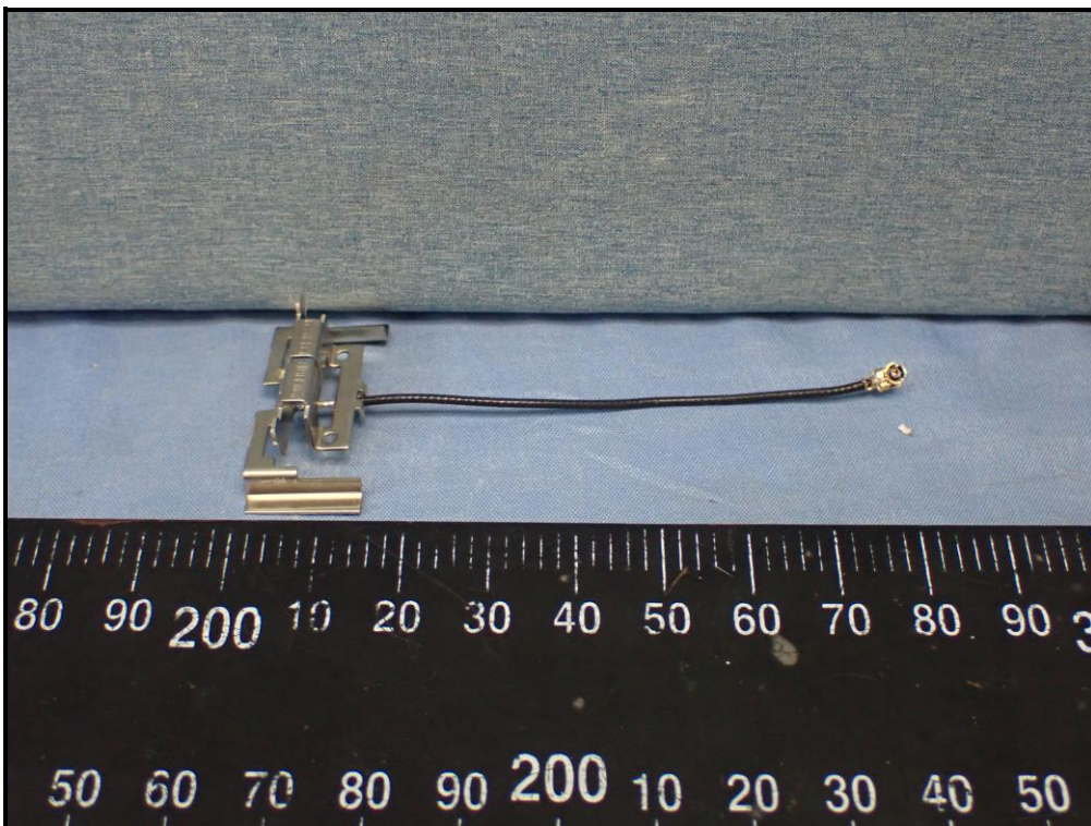
Antenna: 2.4G_0
