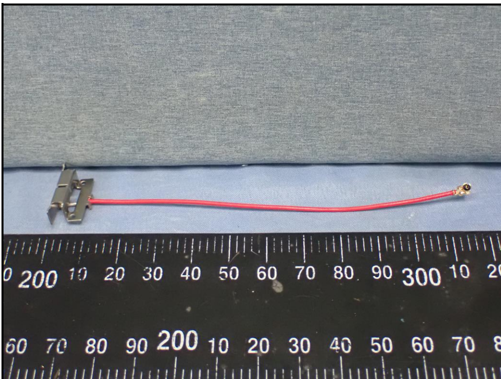
Antenna: 5G_0
