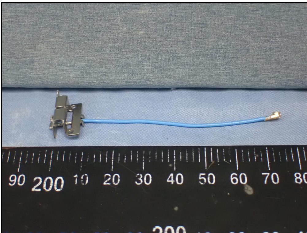
Antenna: 5G_1
