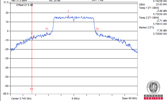
802.11ax (HE20)_Chain 1 / CH149
