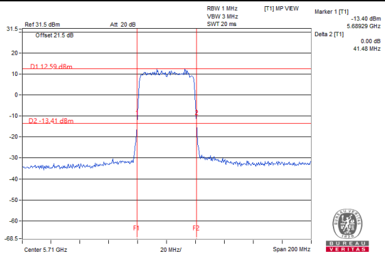
802.11ax (HE40)_Chain 2 / CH142
