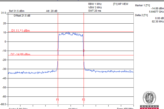
802.11ax (HE80)_Chain 2 / CH138
