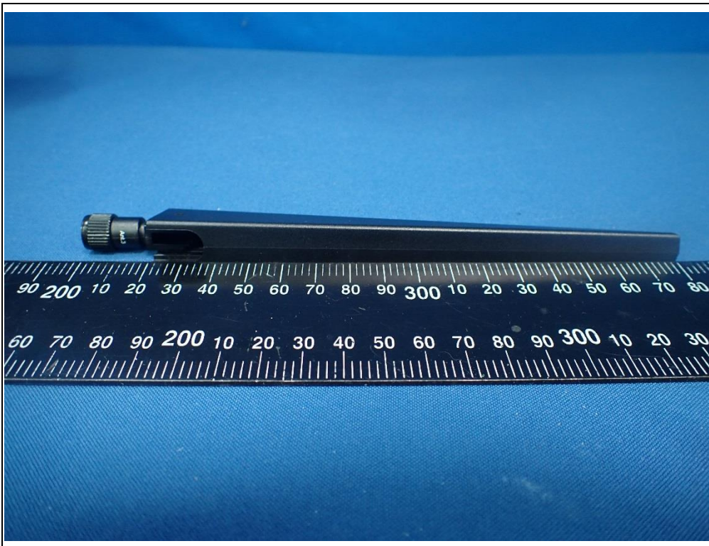
Single_Ant.
