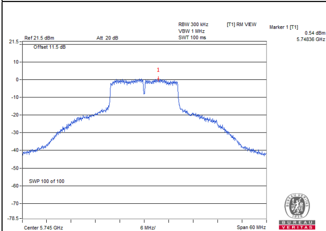
802.11ac (VHT40)
