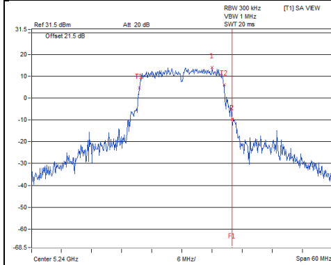
802.11ax (HE20)_Chain 0 / CH48
