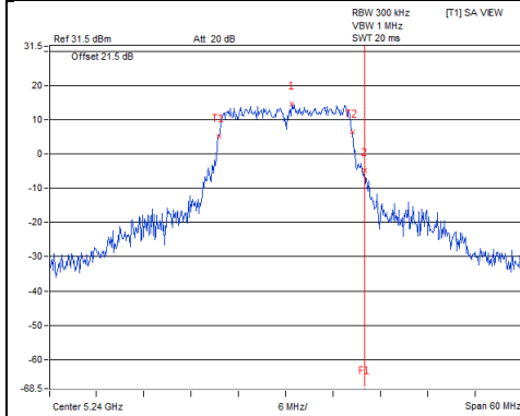
802.11a_Chain 2 / CH48
