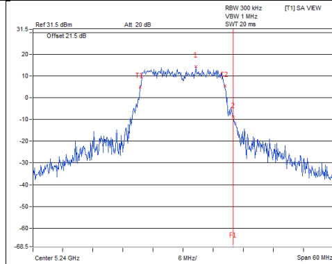
802.11ax (HE20)_Chain 1 / CH48
