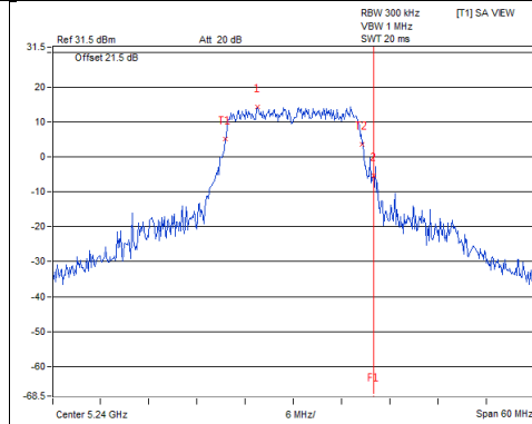
802.11a_Chain 3 / CH48
