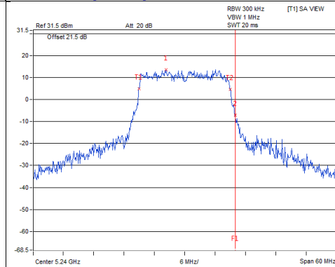
802.11ax (HE20)_Chain 3 / CH48
