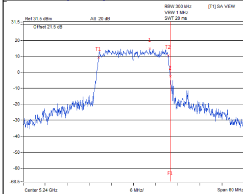
802.11ax (HE20)_Chain 2 / CH48
