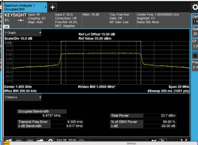
20MHz / QPSK
