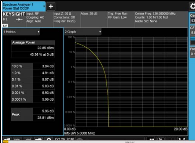
5MHz / 16QAM
