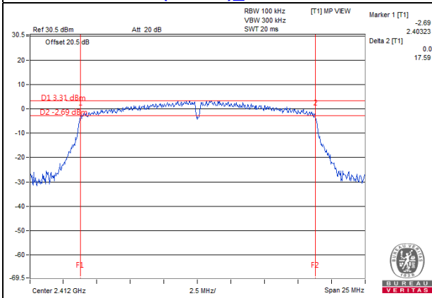
802.11n (20MHz)_Chain 1 / CH 1
