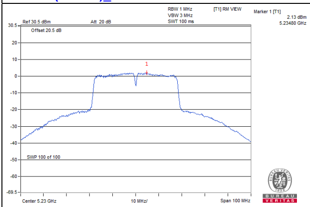
802.11n (40MHz)_Chain 0 / CH 46
