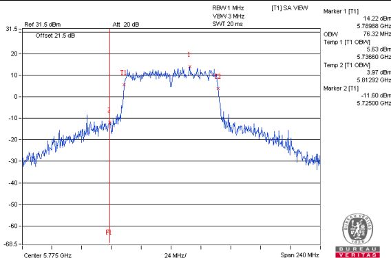
802.11ac(VHT80)_Chain2 / CH155
