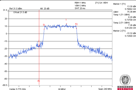
802.11ac(VHT80)_Chain1 / CH155
