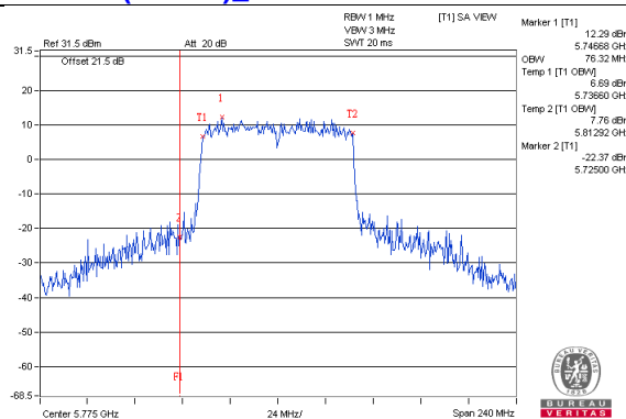
802.11ac(VHT80)_Chain1 / CH155
