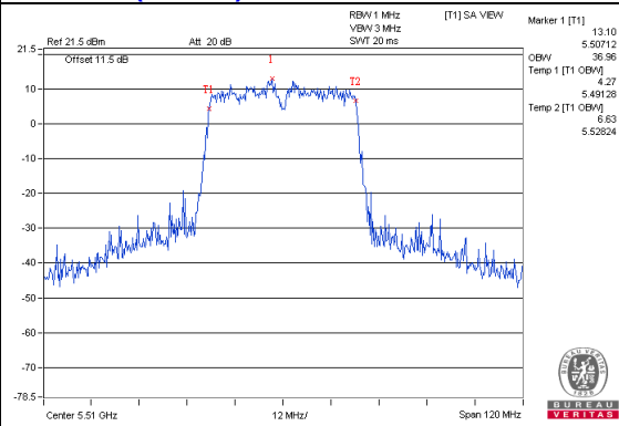
802.11ac (VHT40)_Chain2 / CH102
