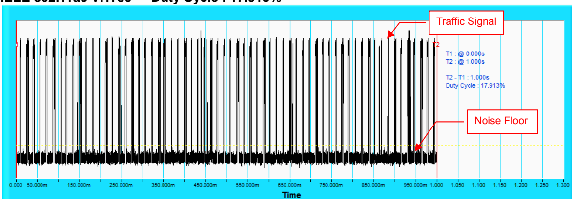
IEEE 802.11ac VHT80 Duty Cycle : 17.913%
